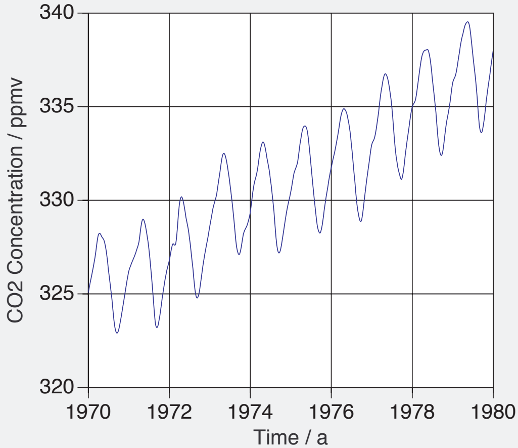
Atmospheric CO2
